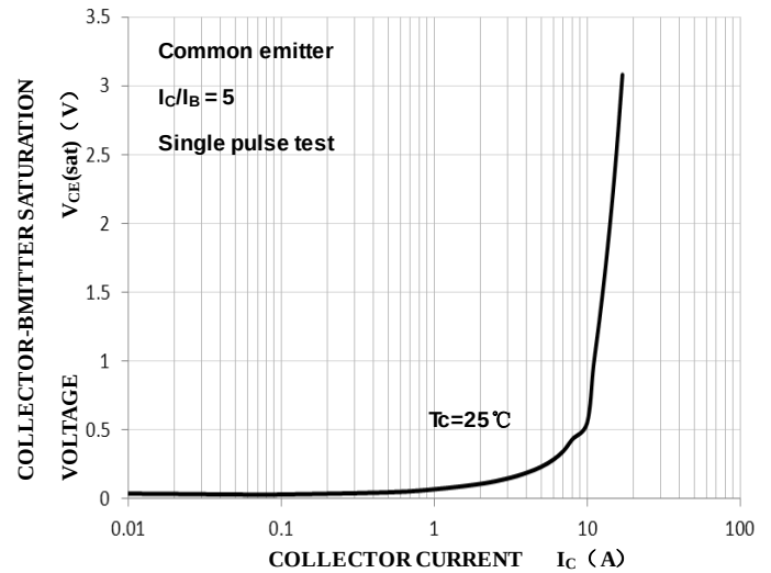
V_{CE(sat)} - I_C (MJL21193)
