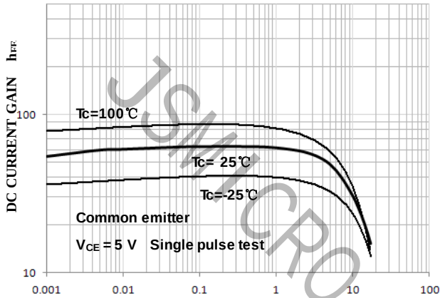
h_{FE} - I_C (MJL21193)
